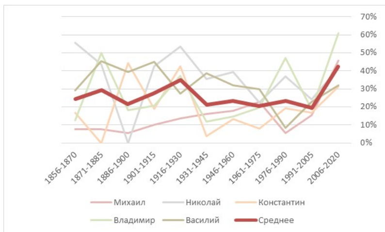
Рис. 3. Средние значения встречаемости полных форм мужских имен, %
