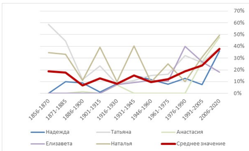
Рис. 4. Средние значения встречаемости полных форм женских имен, %
