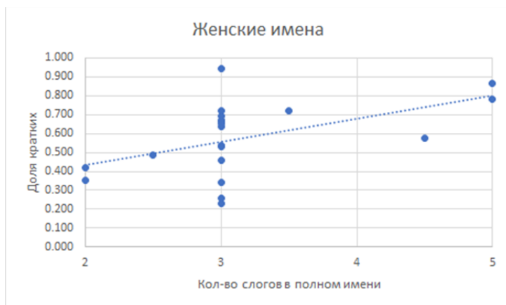
Рис. 2. Зависимость доли кратких имен от числа слогов в женском имени. Коэффициент ранговой корреляции Спирмена \rho = 0,559 ( p = 0,01 )
