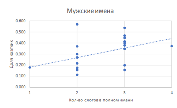
Рис. 1. Зависимость доли кратких имен от числа слогов в мужском имени. Коэффициент ранговой корреляции Спирмена \rho = 0,462 ( p = 0,04 )
