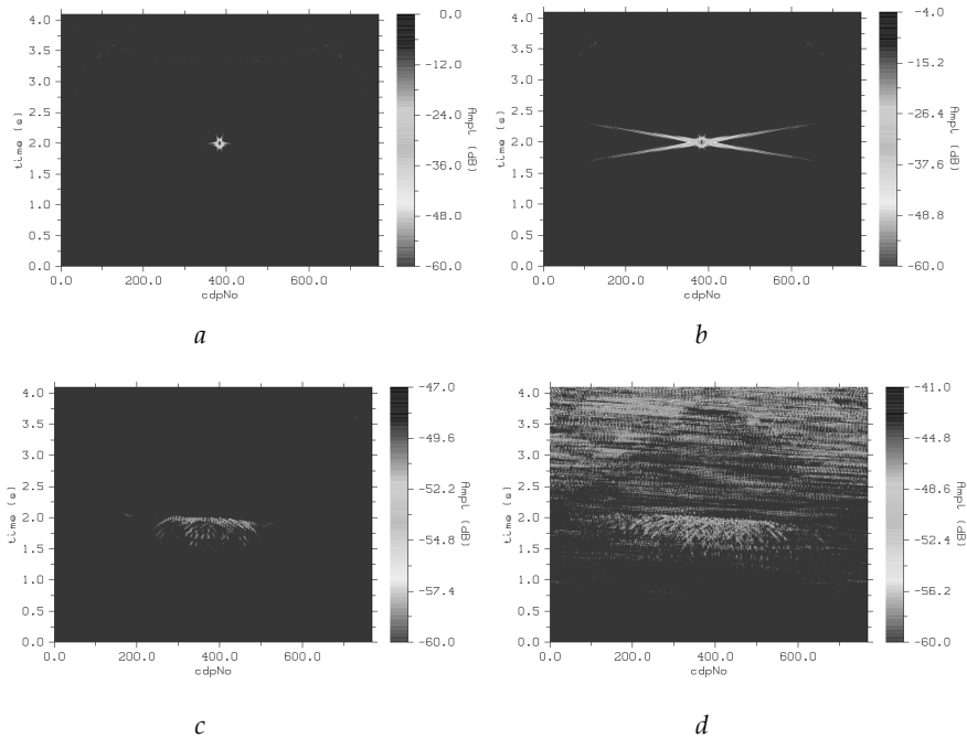
Рис. 1. Логарифмические временные разрезы точечного дифрактора и остатков от рефлектора:
