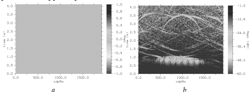
Рис. 2. Результат реконструкции дифрактора, затененного рефлексором. Амплитуда рассеянной волны в 100 раз меньше амплитуды отраженной волны: a – разрез в линейном; b – в логарифмическом масштабах
