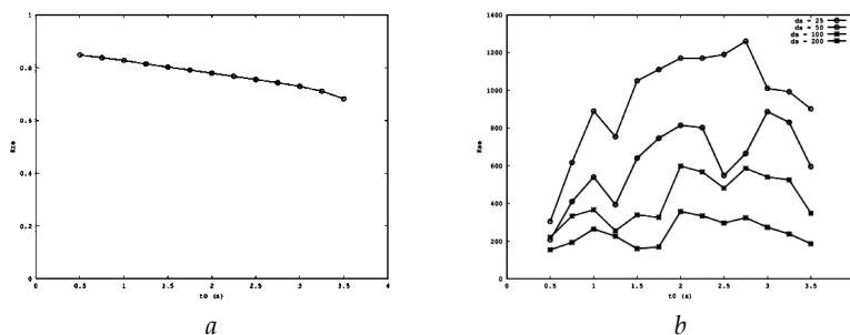
Рис. 3. Зависимость коэффициента реконструкции точечного дифрактора k_{re} от t_0 ( a ) и зависимости коэффициента чувствительности k_{sc} от t_0 для различных значения \Delta s ( b )
